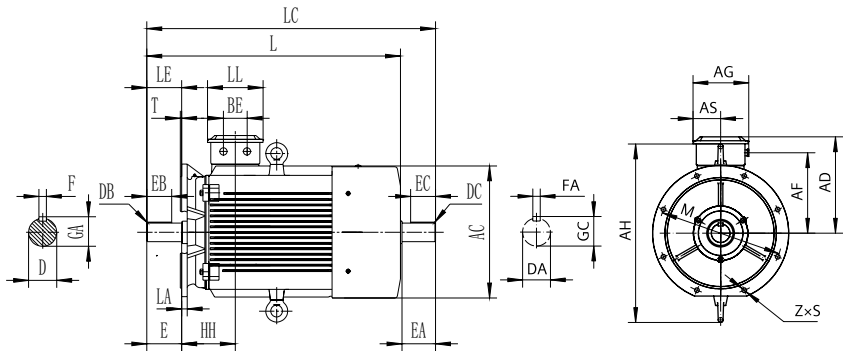
IM B14 安装结构型式 Type of construction IM B14
